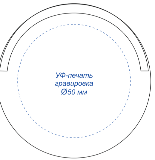
Крышка
